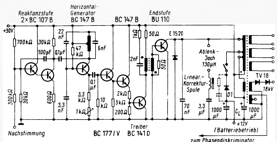
Bild 1. Niederspannungsschaltung zur Horizontalablenkung
