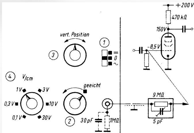
Bild 6. Benützung eines Oszillografen für Gleichspannungsmessungen
