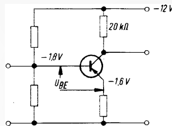
Bild 2. Betriebsverhalten eines Transistors in Abhängigkeit von der Betriebsspannung
