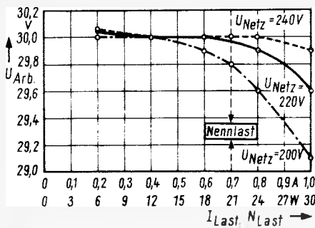
Links: Bild 5. Arbeitsspannung in Schaltung I (Bild 3). Abhängigkeit von Belastung und Netzspannung
