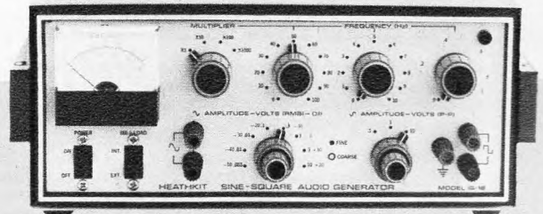
Sinus-Rechteckgenerator IG-18
