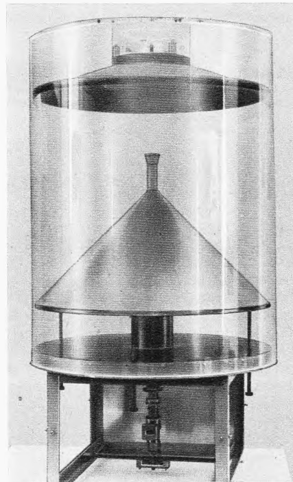
Bild 3. Rundstrahlantenne mit kreisförmiger Horizontalcharakteristik (Gewinn: 8...10 dB, Halbwertswinkel der Vertikalcharakteristik \approx 5^\circ )
