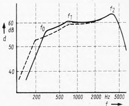
Bild 3. Ideale Frequenzkurve eines Kleinlautsprechers
