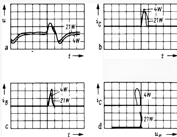
Bild 7. Oszillogramme zur Pumptransistorschaltung II: a = Basisspannung des Pumptransistortreibers, b = Basisstrom und c = Kollektorstrom des Pumptransistors, d = Arbeitskennlinie des Pumptransistors
