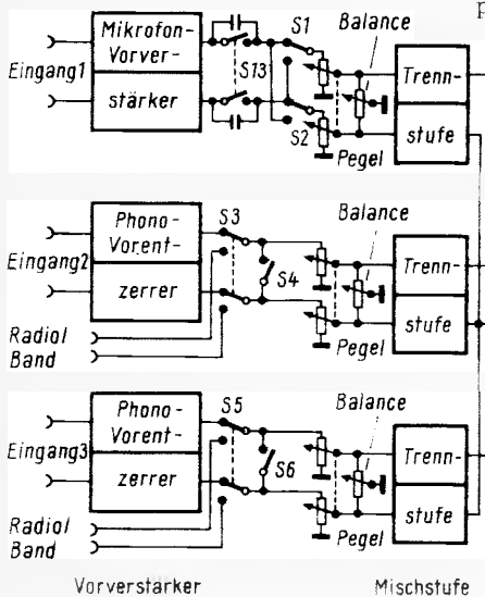
Bild 1. Blockschaltung des Mischpultverstärkers
