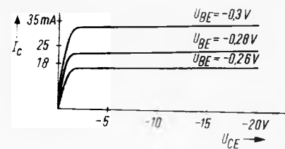
Bild 2. Betriebsverhalten eines Transistors in Abhängigkeit von der Betriebsspannung
