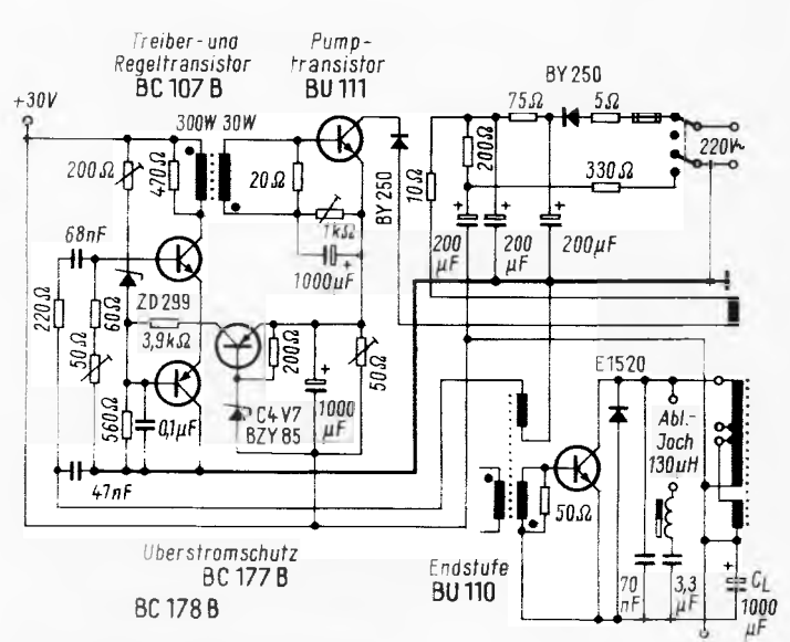
Bild 4. Pumptransistorschaltung II (mit Überstromschutz)
