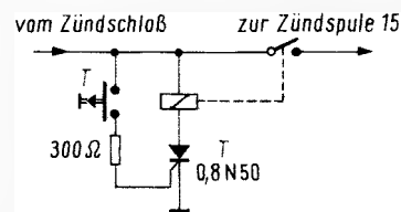
Einfache Schaltung einer Diebstahlsicherung für eine 6-V-Anlage
