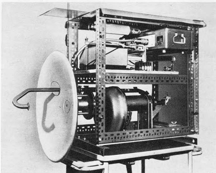
Bild 6. Der Mikrowellen-Meßempfänger auf der Spitze des Mastes des Beobachtungswagens. Links der Parabolspiegel (65 cm \varnothing ) mit Einspeisung durch einen Rechteckhohlleiter, rechts daneben Getriebe und Motor zum Drehen der Polarisationssebene. Darüber der Empfänger mit Oszillator (links), Mischer und Nachverstärker (Mitte); oben rechts das Steuergerät mit Verstärker und Netzteil für die Fernsehkamera (ganz oben in dem röhrenförmigen Gehäuse), die zum Ausrichten des Parabolspiegels auf die Sendeantenne dient
