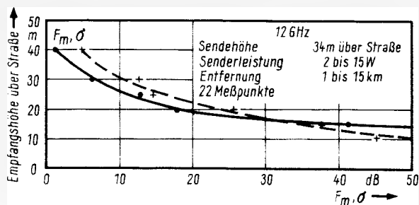
Links: Bild 7. Feldstärke in Abhängigkeit von der Höhe über Straßenniveau
