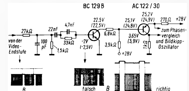
Schaltung des Amplitudensiebes. Durch den zu geringen Sperrwiderstand der Basis-Emitter-Strecke des Transistors BC 129 B wurden die Bild-Synchronimpulse abgeschnitten
